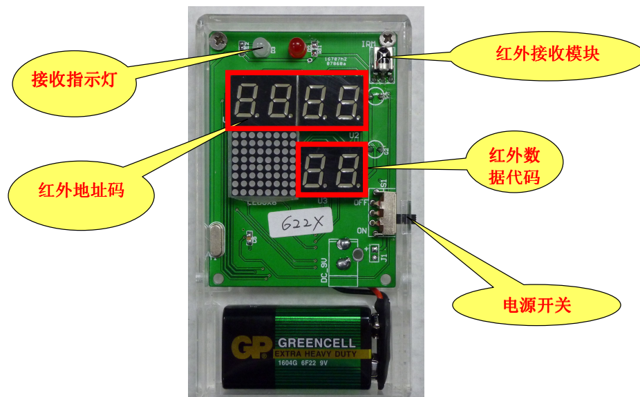
图 2：红外接收器
