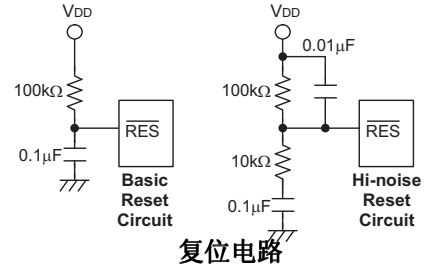
注: 在一般应用场合可使用基本复位电路, 而在强干扰环境中, 建议使用抗杂讯复位电路。
