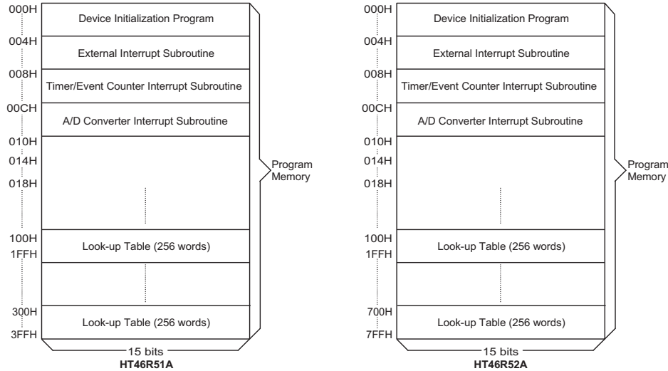
程序存储器
