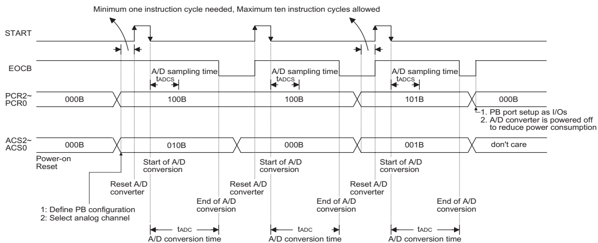
A/D 转换时序
