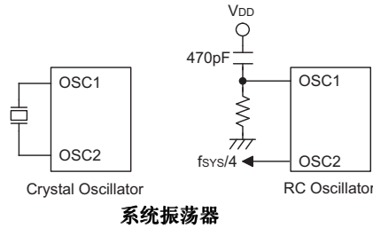
系统振荡器
