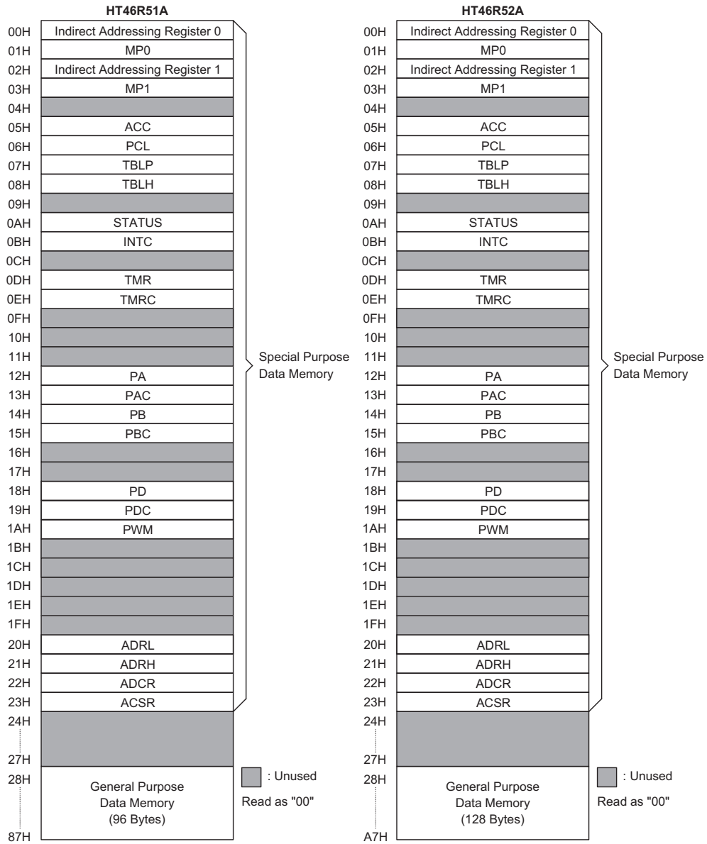
数据存储器
