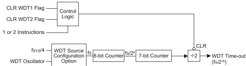
看门狗定时器
