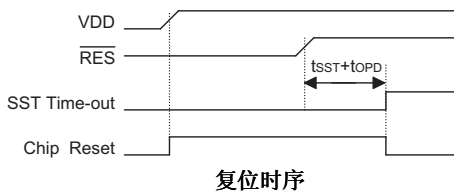
复位时序
