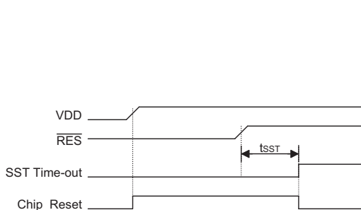
复位时序图
