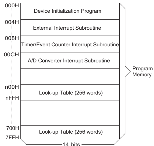
HT46R47/HT46C47 程序存储器
