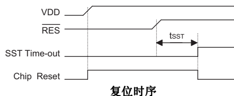
复位时序
