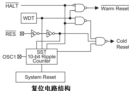
复位电路结构
