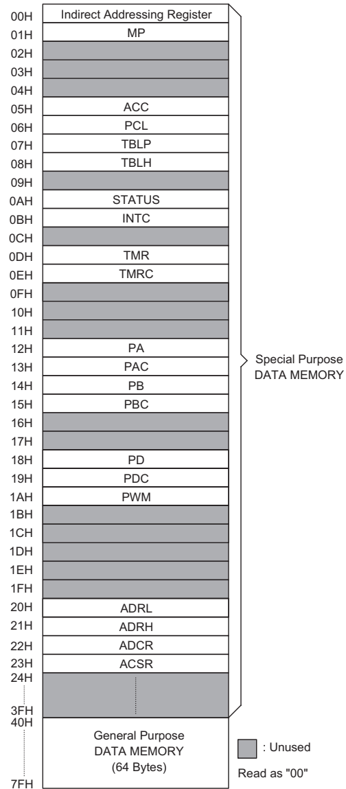
HT46R47/HT46C47 的数据存储器
