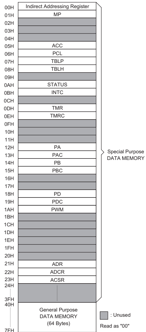
HT46R46/HT46C46 的数据存储器
