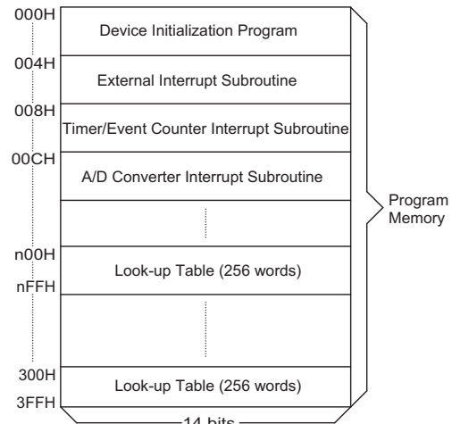
HT46R46/HT46C46 程序存储器
