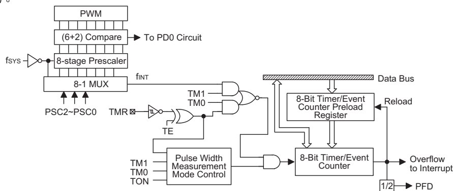
定时/计数器
