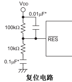
复位电路
