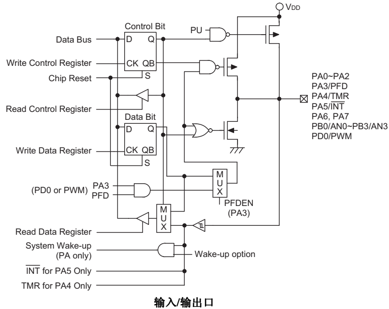
输入/输出口
