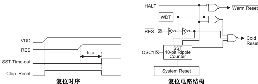
复位时序
