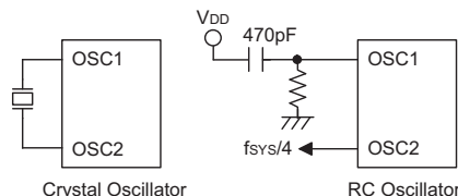
系统振荡器
