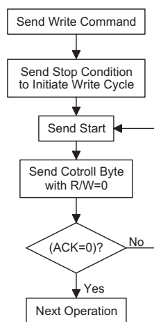
检测应答信号流程
