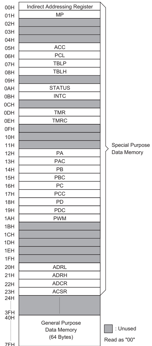
数据存储器
