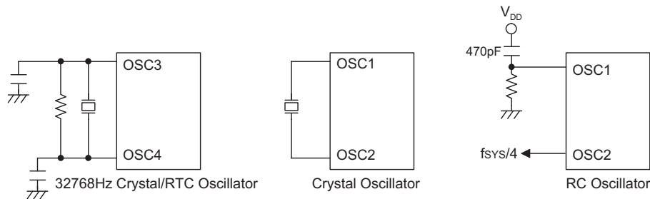
系统振荡器
