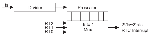
实时时钟
