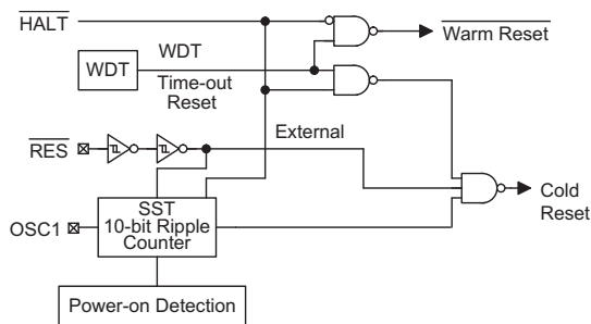
复位配置
