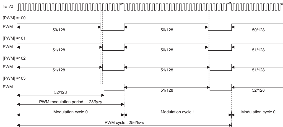
(7+1)位模式 PWM
