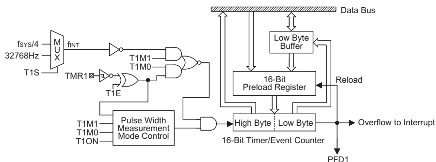
定时/计数器 1
