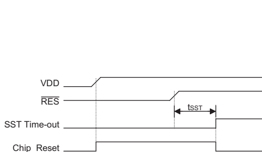
复位时序图
