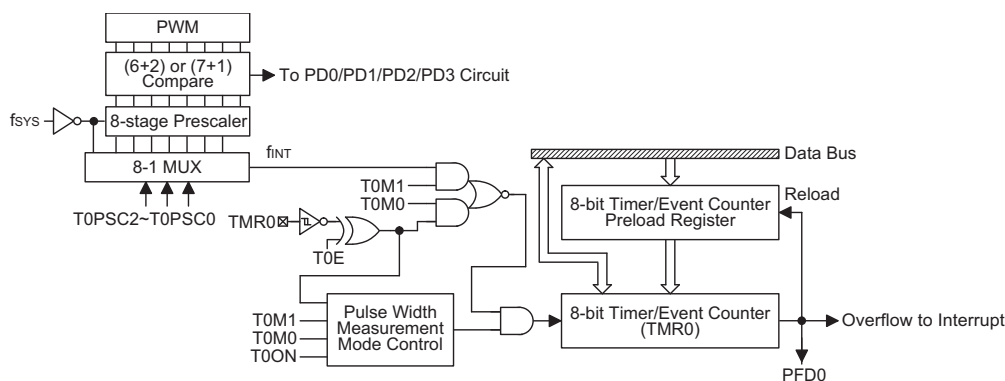
定时/计数器 0
