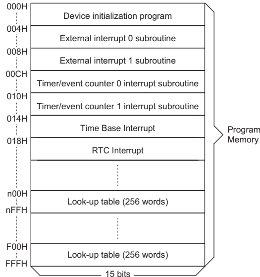
程序存储器
