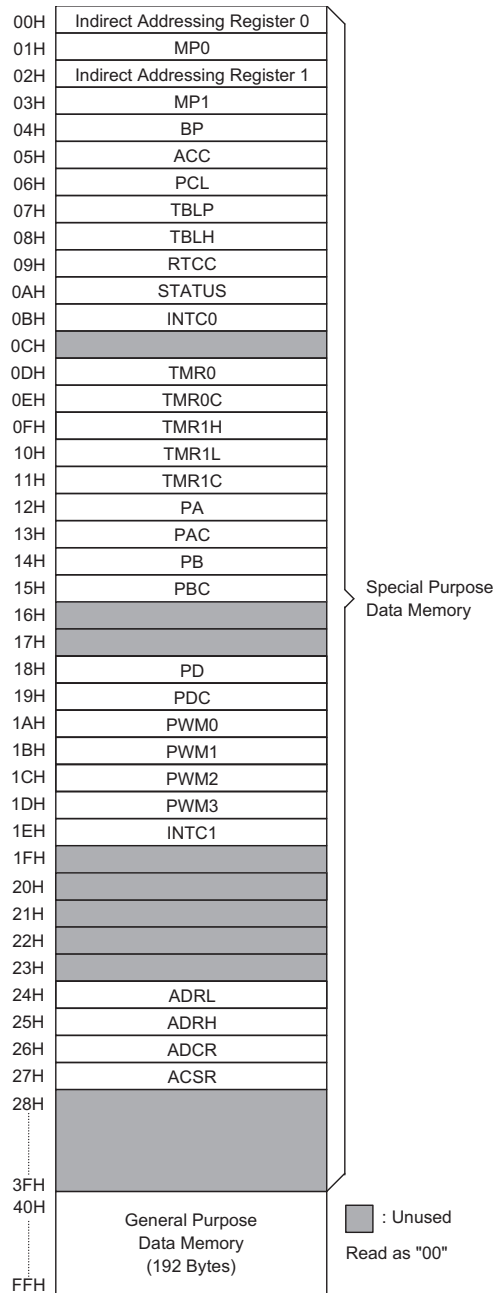
数据存储器
