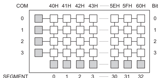
显示存储器
