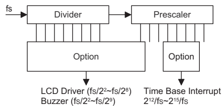
时基
