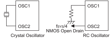
系统振荡器
