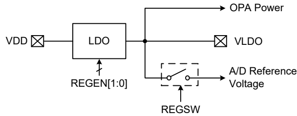
LDO 方框图
