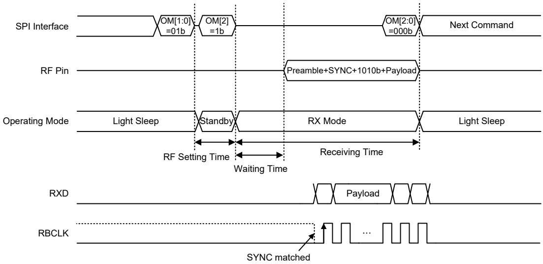
Direct 模式 RX 时序图
