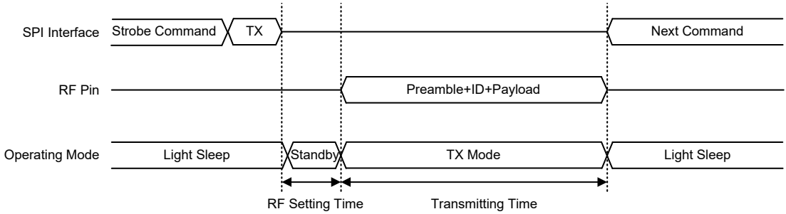
FIFO 模式 TX 时序图
