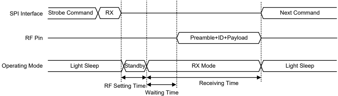
FIFO 模式 RX 时序图
