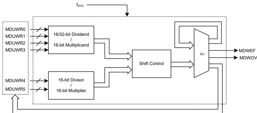
16-bit MDU 方框图
