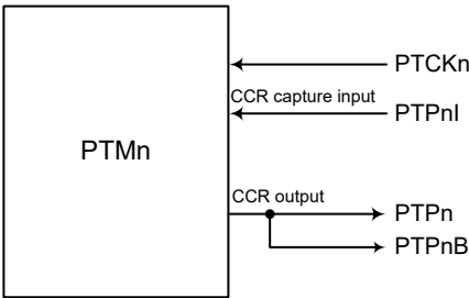
PTM 功能引脚控制方框图 (n=0)
