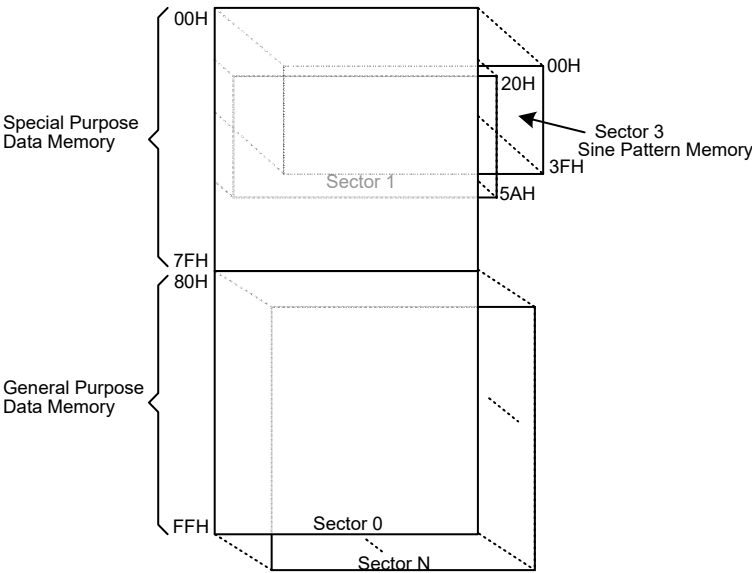
注：对于 BH66F2650, N=1；对于 BH66F2660, N=7 数据存储器结构
