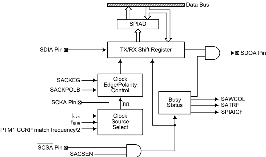
SPIA 方框图
