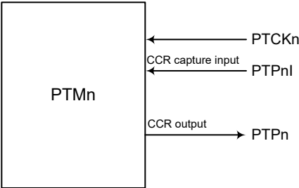
PTM 功能引脚控制方框图 (n=1, 2)
