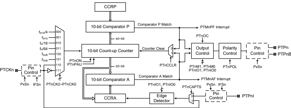
周期型 TM 方框图 (n=0, 1, 2)
