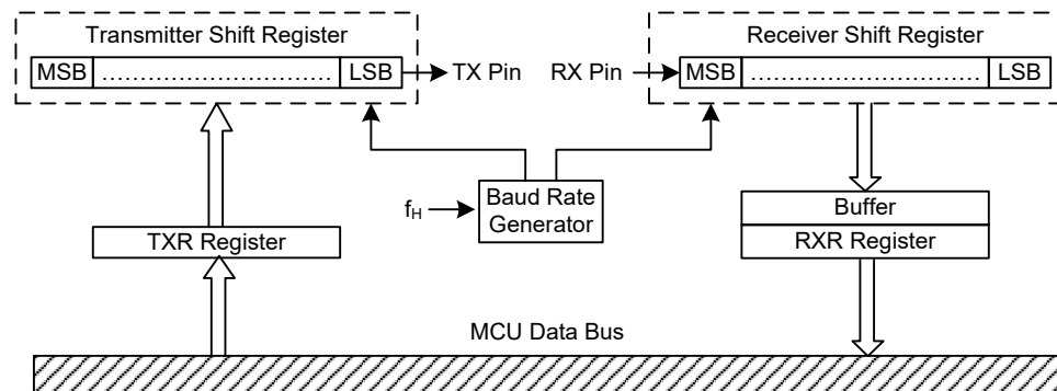
UART 数据传输方框图
