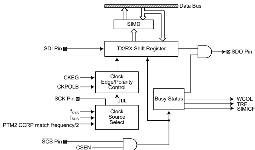
SPI 方框图
