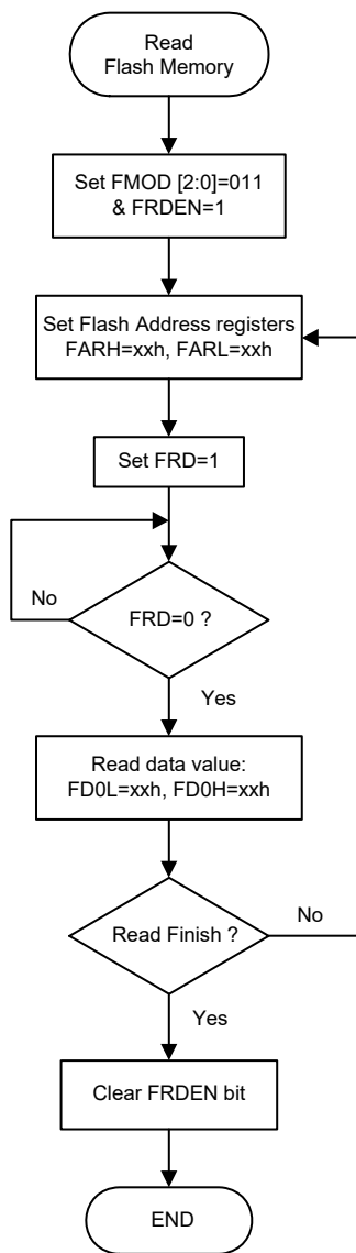
读 Flash 程序存储器步骤
