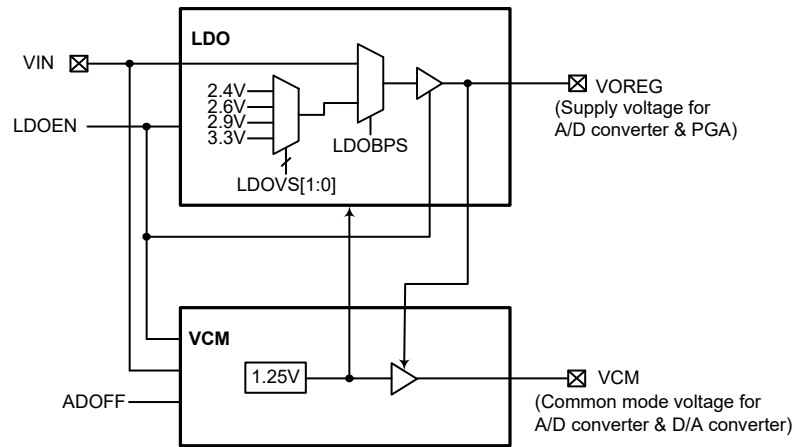
内部电源供电方框图
