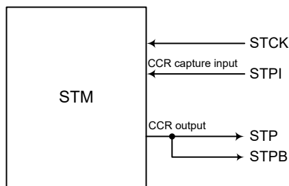
STM 功能引脚控制方框图
