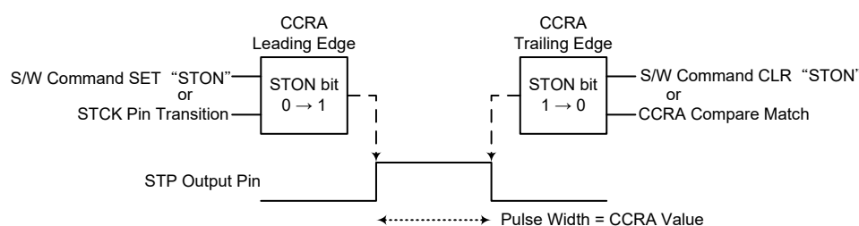
单脉冲产生示意图
