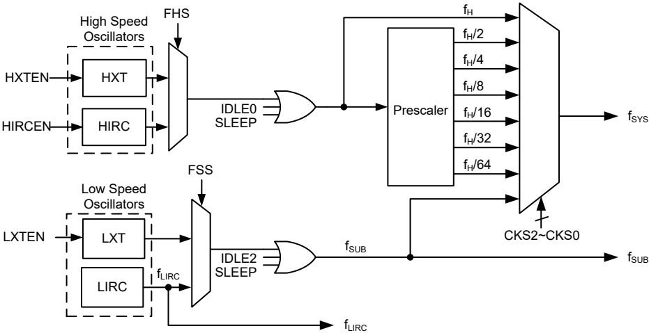
系统时钟配置
