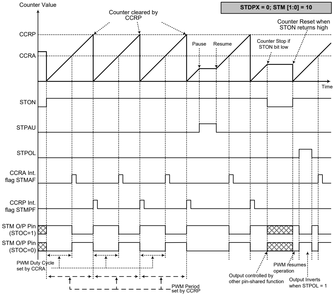
PWM 输出模式 – STDPX=0
