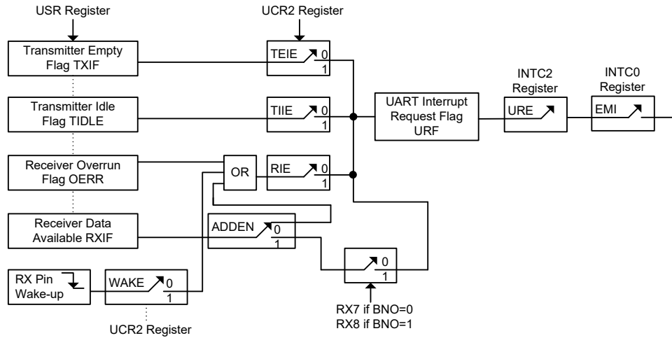
UART 中断结构
