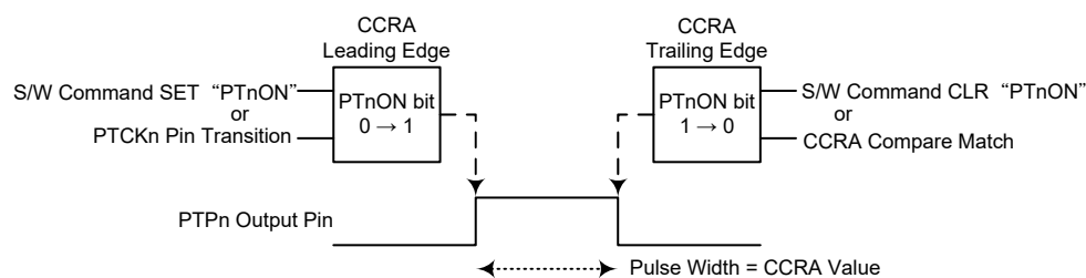
单脉冲产生示意图 (n=0, 1, 2)
