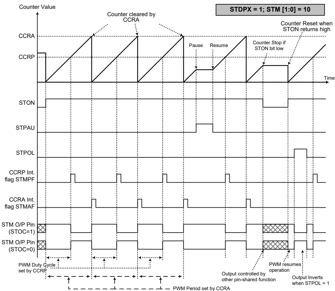
PWM 输出模式 – STDPX=1
