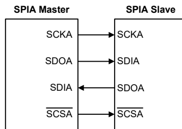
SPIA 主 / 从机连接方式
