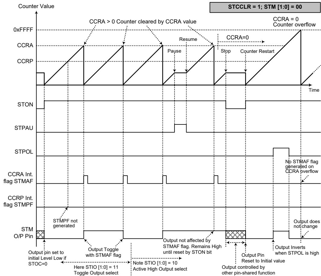
比较匹配输出模式 – STCCLR=1
