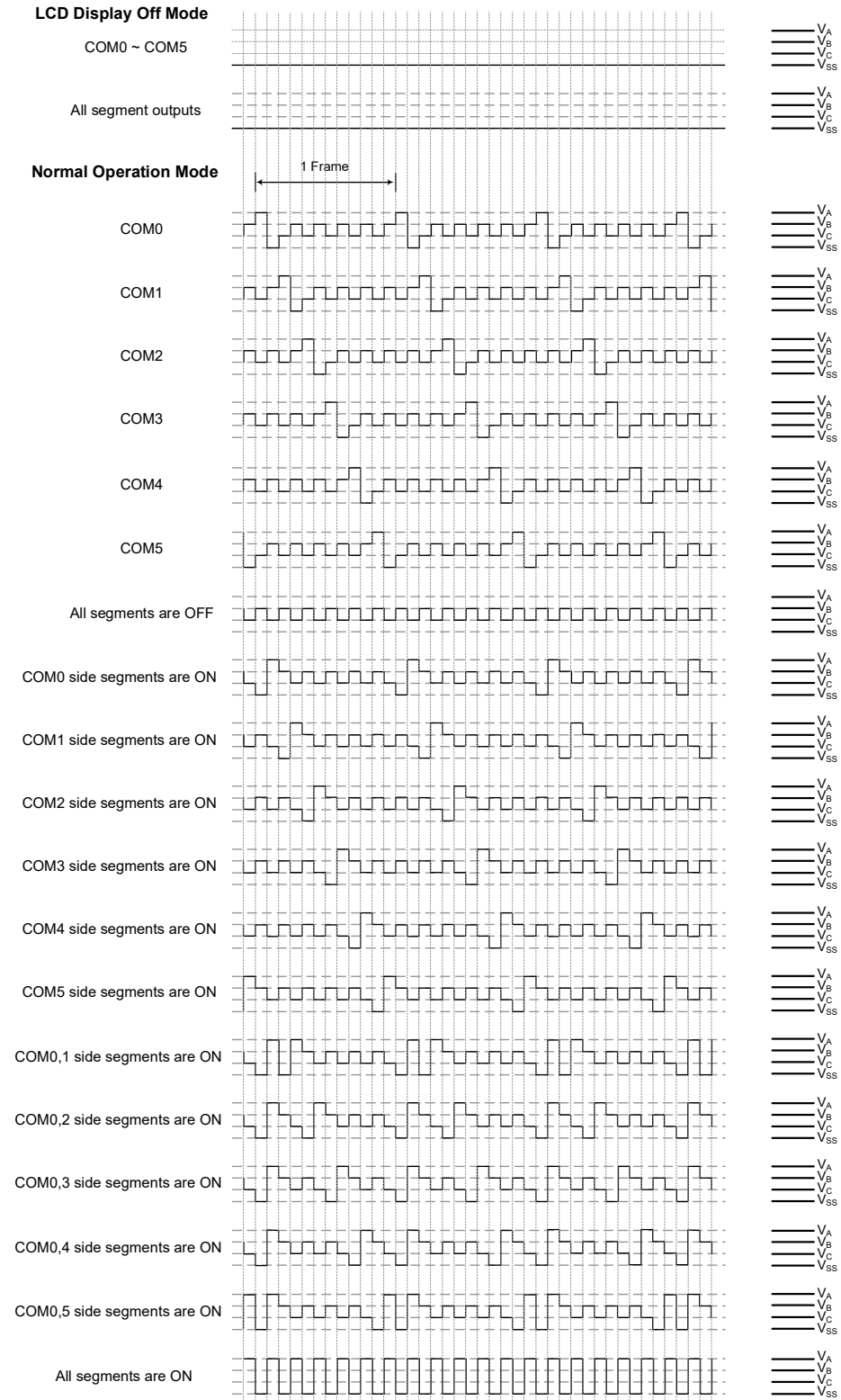
LCD 驱动输出 – A 型, 1/6 Duty, 1/3 Bias
