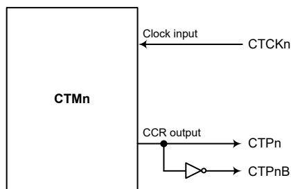
CTMn 功能引脚方框图 (n=0~1)
