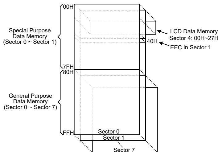
数据存储器结构
