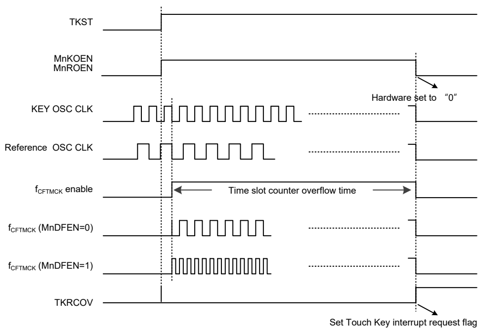
触控按键时序图
