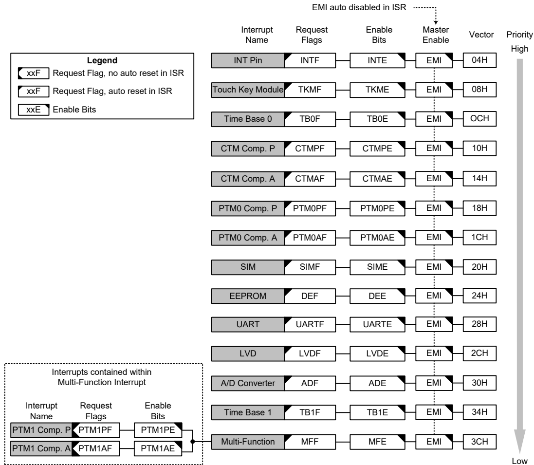
中断结构
