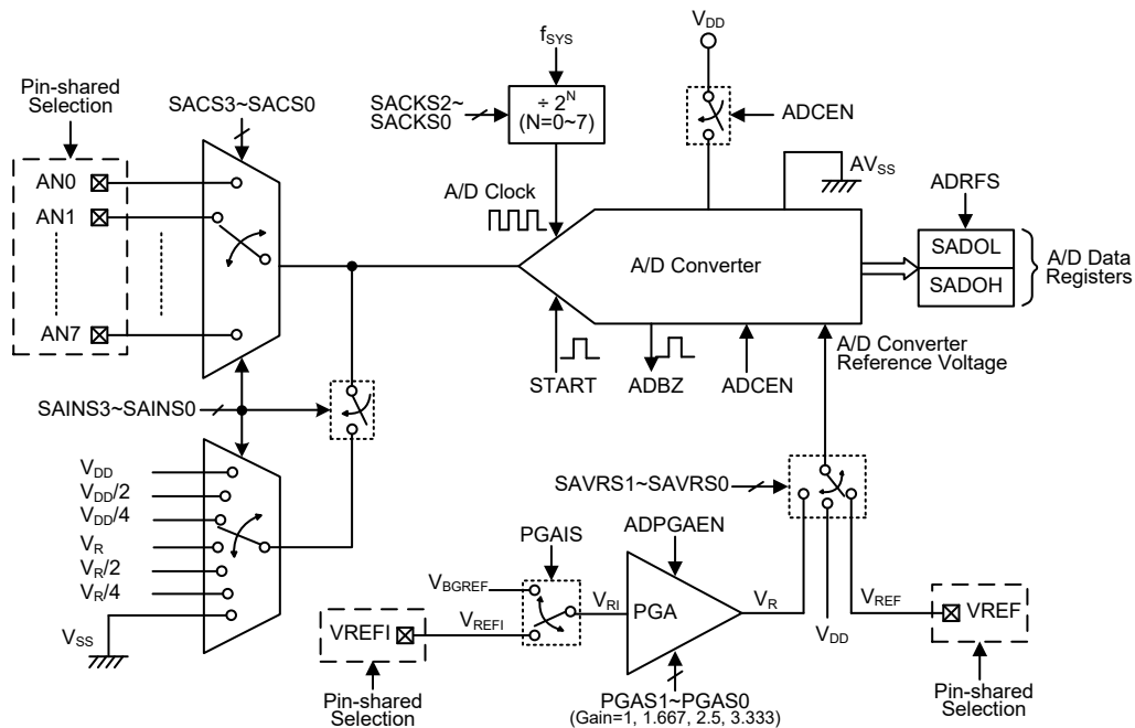
A/D 转换器结构
