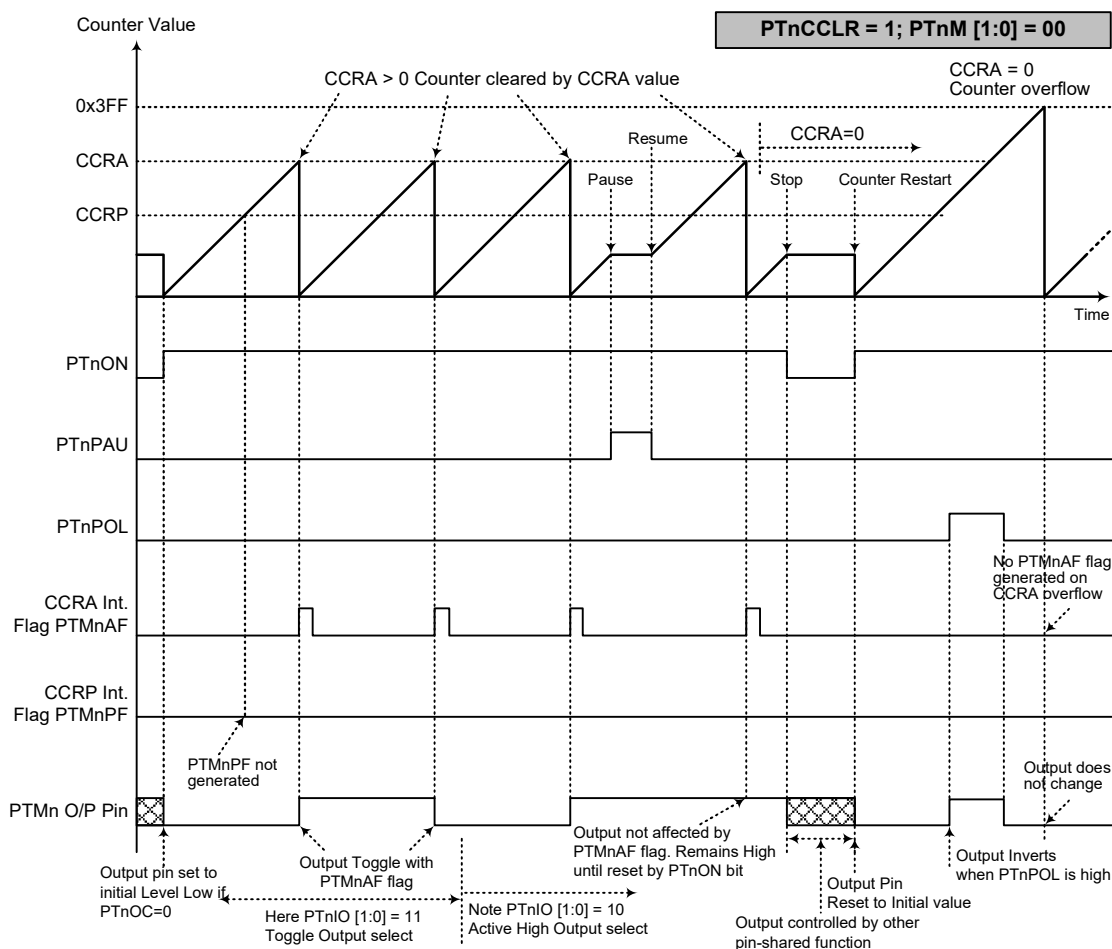
比较器匹配输出模式 – PTnCCLR=1 (n=0~1)
