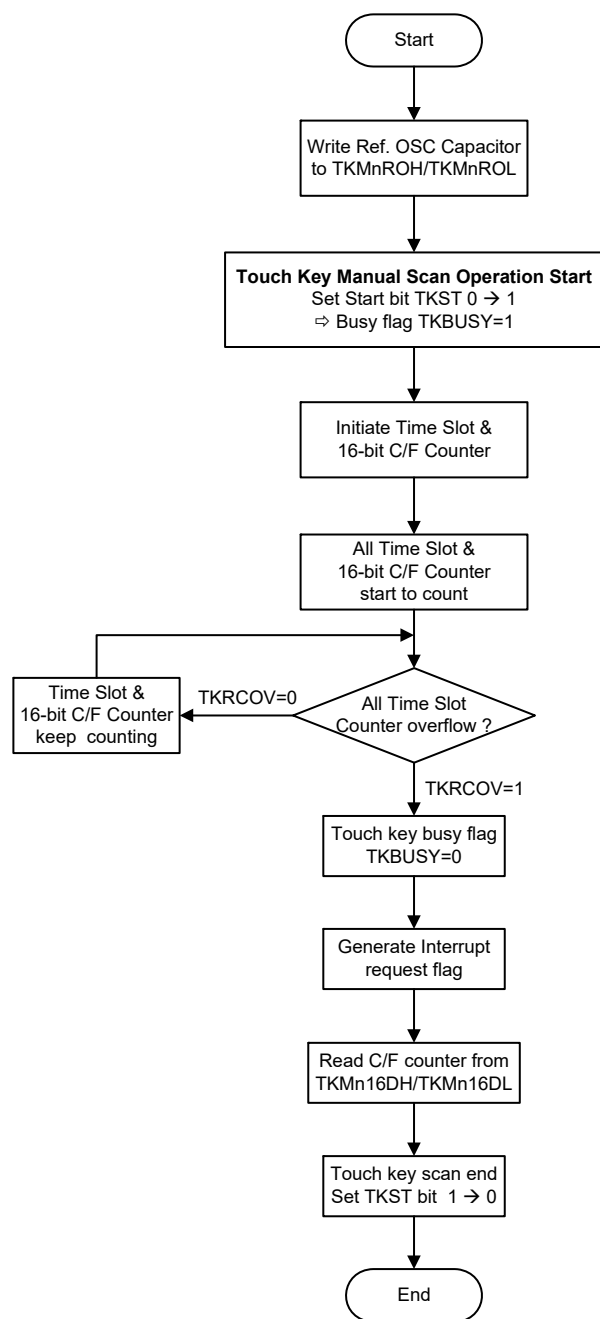
手动扫描模式流程图 – TKMOD=1, TSCS=0
