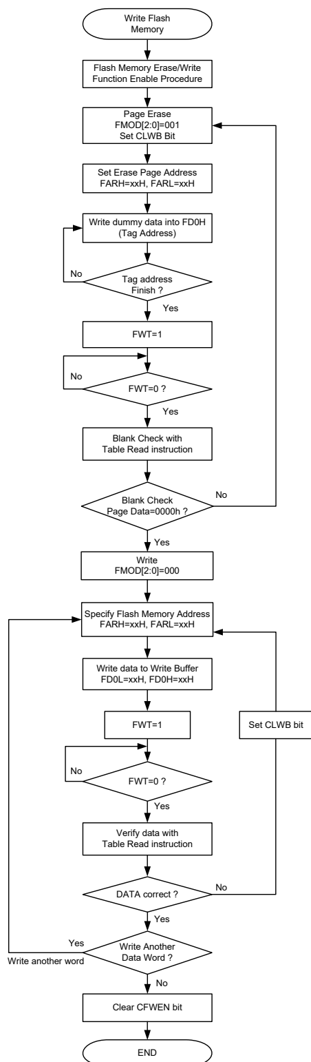
Flash 存储器非连续地址写入程序
