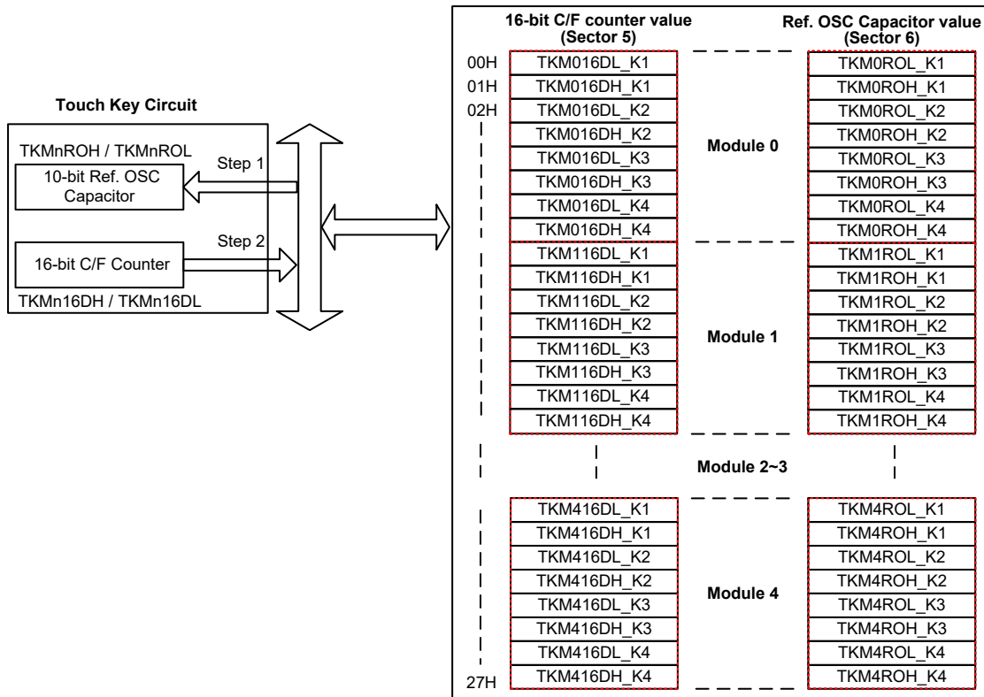
触控按键模块数据存储区分布
