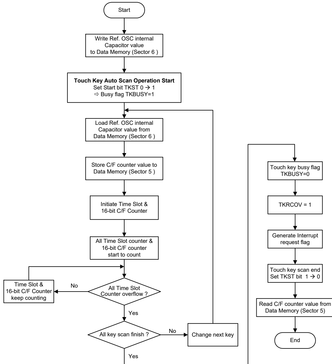
自动扫描模式流程图 – TKMOD=0, TSCS=0
