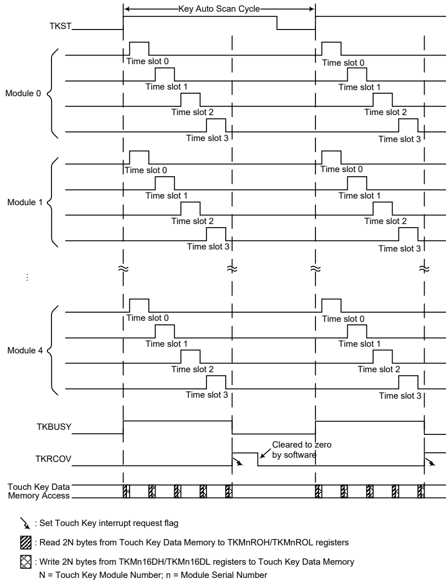
触控按键自动扫描时序图
