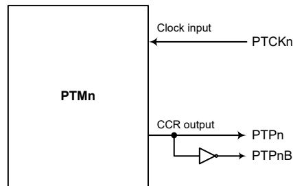
PTMn 功能引脚方框图 (n=0~1)
