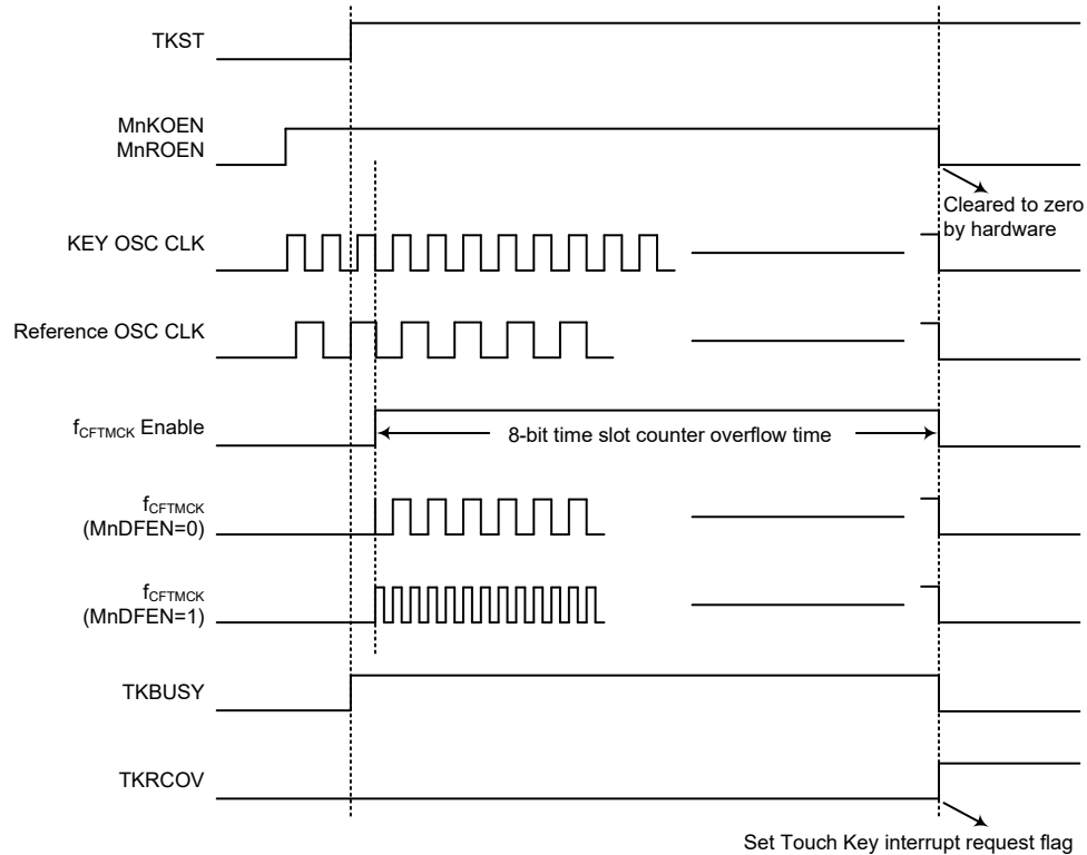
触控按键手动扫描模式时序图
