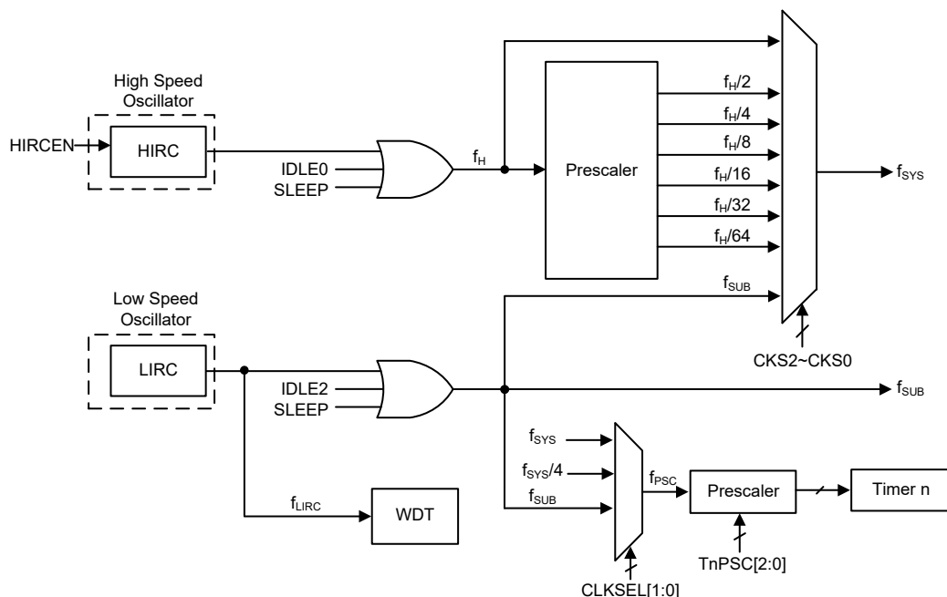
单片机时钟配置
