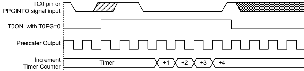
脉冲宽度测量模式的时序图 (T0EG=0)
