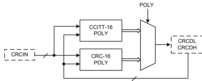
CRC 方框图
