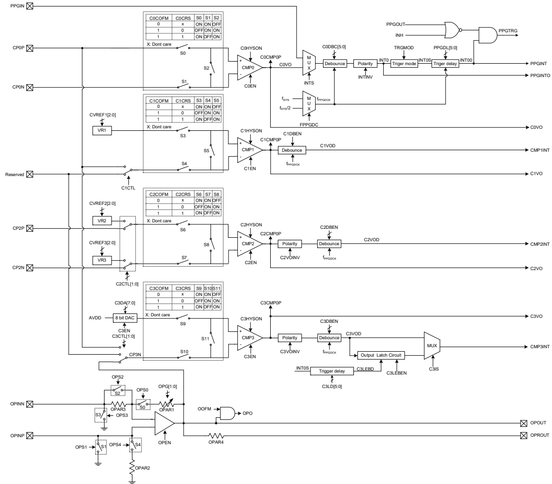
比较器 & 运算放大器方框图
