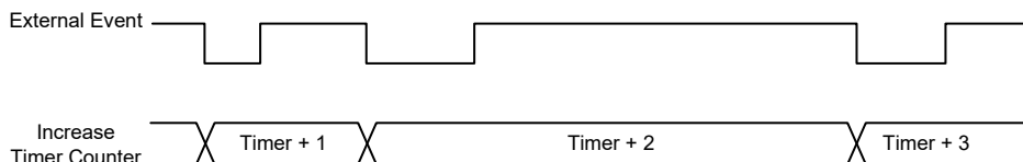
事件计数器模式时序图 (TEG=1)
