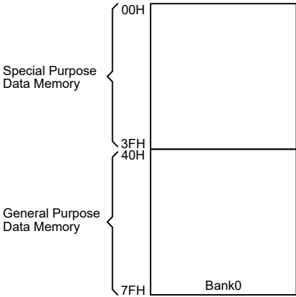
数据存储器结构
