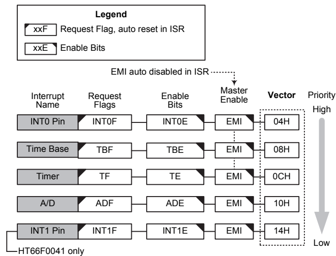
中断结构
