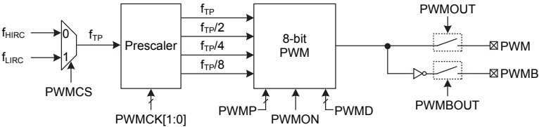
PWM 方框图
