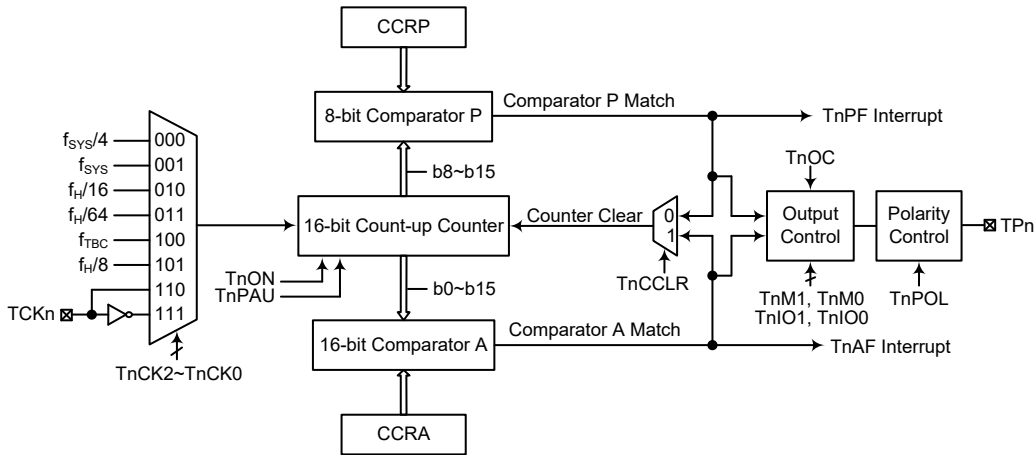
简易型 TM 方框图 (n=2)
