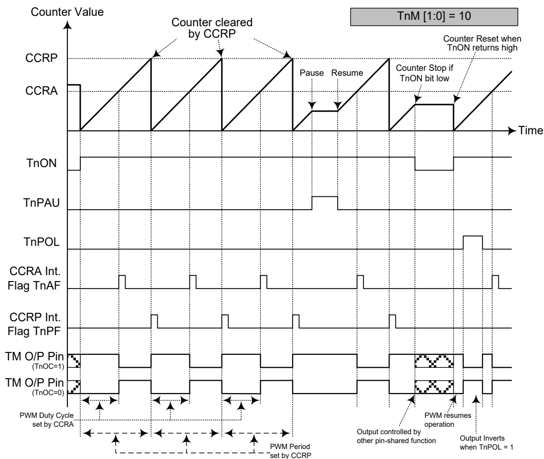
PWM 模式 (n=1)
