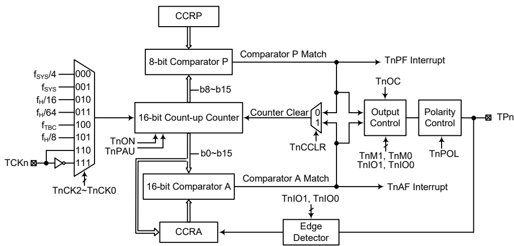
标准型 TM 框图 (n=0)
