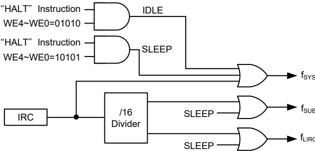
系统时钟配置 – HT68F0012
