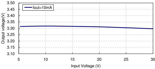
输出电压与输入电压：HT7133-1
