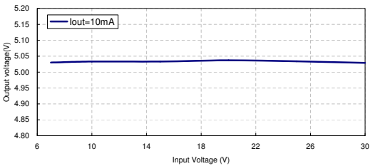
输出电压与输入电压：HT7150-1
