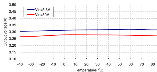
输出电压与温度: HT7133-1
