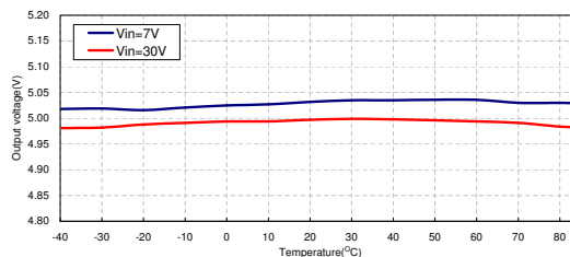
输出电压与温度: HT7150-1
