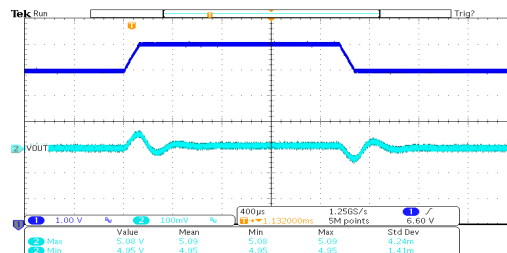
线性瞬态响应: HT7150-1 ( V_{IN}=6V \sim 7V , I_{OUT}=10mA )
