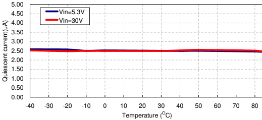
静态电流与温度：HT7133-1 (I OUT =0mA)
