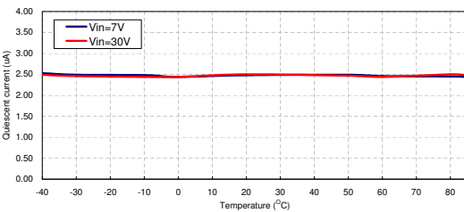
静态电流与温度：HT7150-1 (I OUT =0mA)
