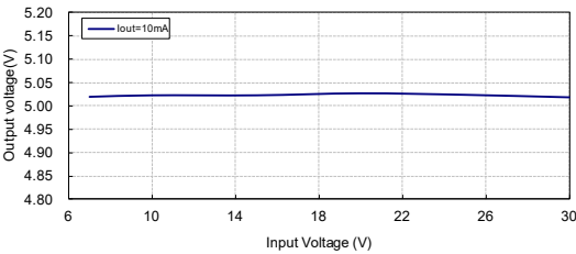
输出电压与输入电压：HT7150-2
