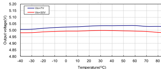
输出电压与温度: HT7150-2
