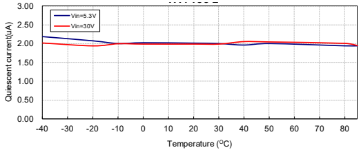
静态电流与温度：HT7133-2 (I OUT =0mA)
