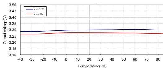
输出电压与温度: HT7133-2
