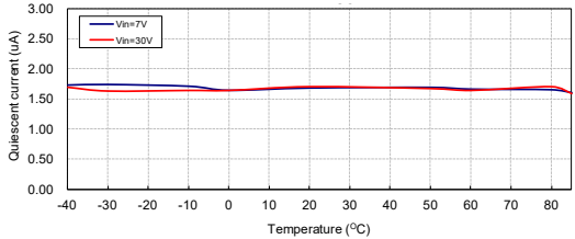
静态电流与温度：HT7150-2 (I OUT =0mA)
