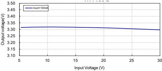
输出电压与输入电压：HT7133-2
