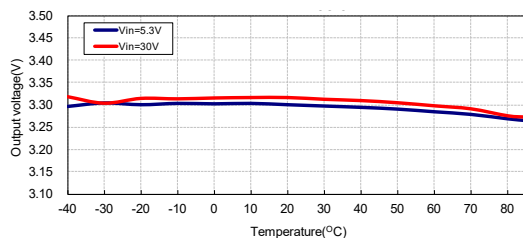
输出电压与温度: HT7133-3
