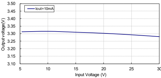
输出电压与输入电压：HT7133-3
