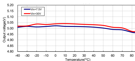
输出电压与温度: HT7150-3
