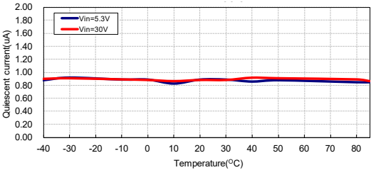
静态电流与温度：HT7133-3 (I OUT =0mA)
