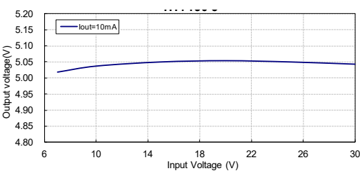
输出电压与输入电压：HT7150-3
