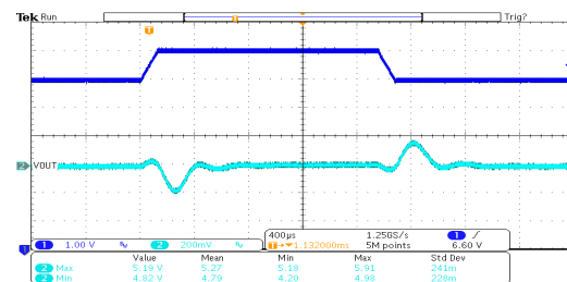
线性瞬态响应: HT7150-3 ( V_{IN}=6V \sim 7V , I_{OUT}=10mA )
