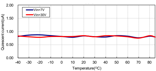
静态电流与温度：HT7150-3 (I OUT =0mA)
