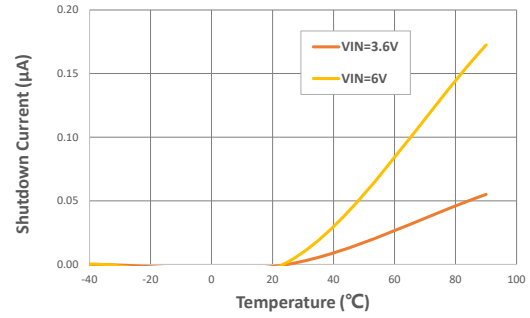
关机电流 vs. 温度
