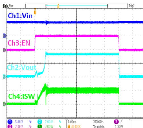
芯片使能 / 除能 ( I_{OUT}=2A )
