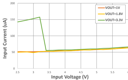
无负载电流 vs. 输入电压
