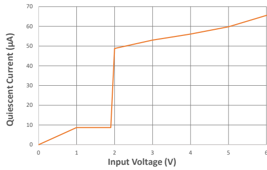
PFM 静态电流 vs. 输入电压
