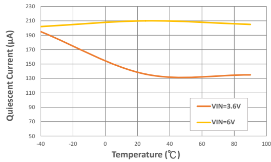
PWM 静态电流 vs. 温度
