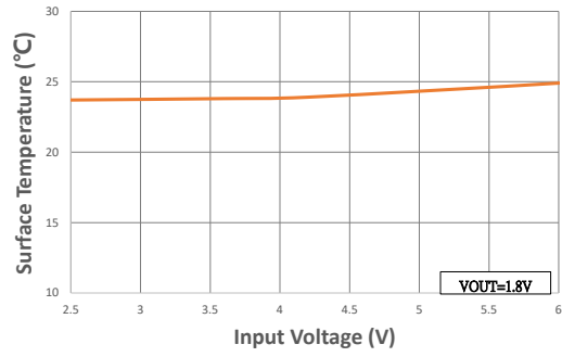
输出短路 表面温度 vs. 输入电压 (8SOP-EP)
