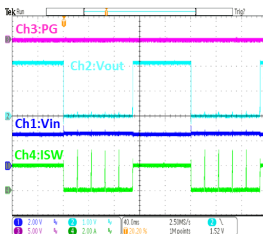
输出短路保护 / 恢复 ( V_{IN}=2.5V , I_{OUT}=2A )
