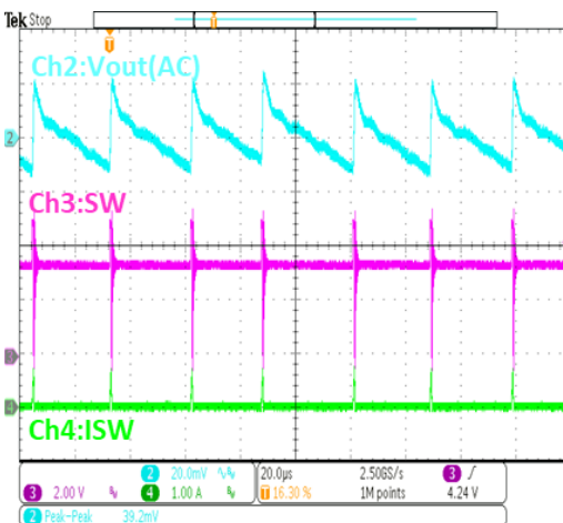
输出纹波 ( I_{OUT}=10mA )
