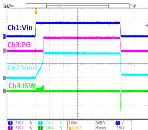
电源上电 / 掉电 ( 空载 )
