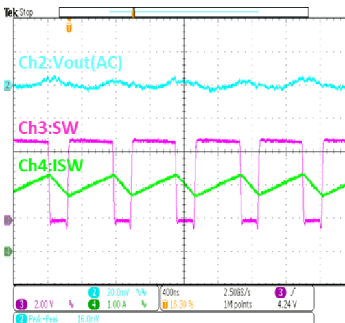
输出纹波 ( I_{OUT}=2A )
