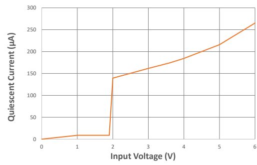
PWM 静态电流 vs. 输入电压
