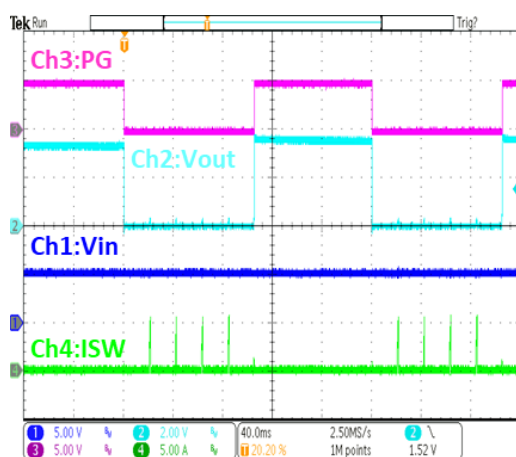
输出短路保护 / 恢复 ( V_{IN}=5V )
