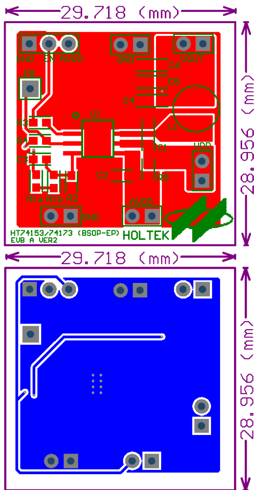
8-pin SOP-EP PCB 布局范例
