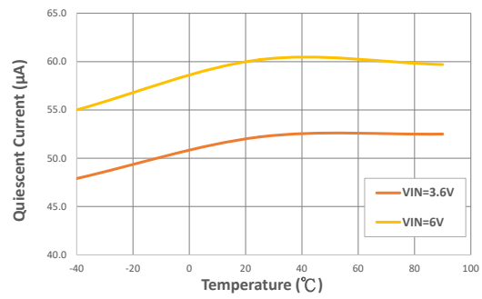
PFM 静态电流 vs. 温度
