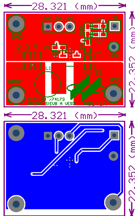
5-pin SOT23 PCB 布局范例
