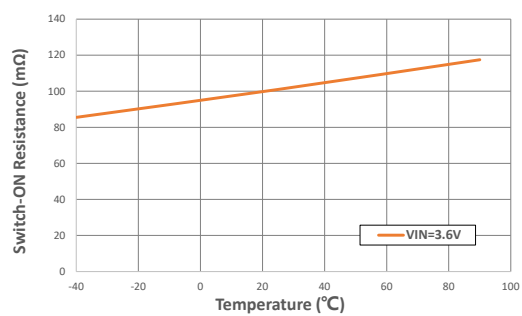
PMOS 导通电阻 vs. 温度
