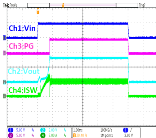
电源上电 / 掉电 ( I_{OUT}=2A )
