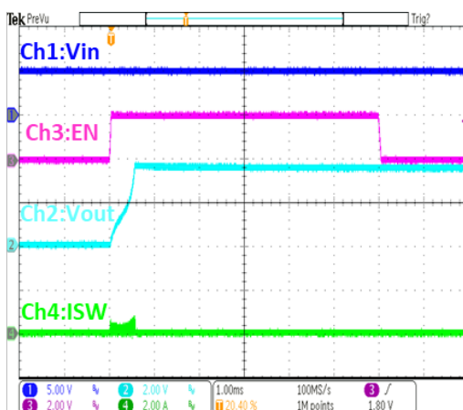
芯片使能 / 除能 ( 空载 )
