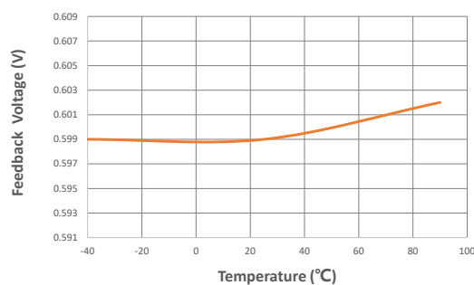
反馈电压 vs. 温度
