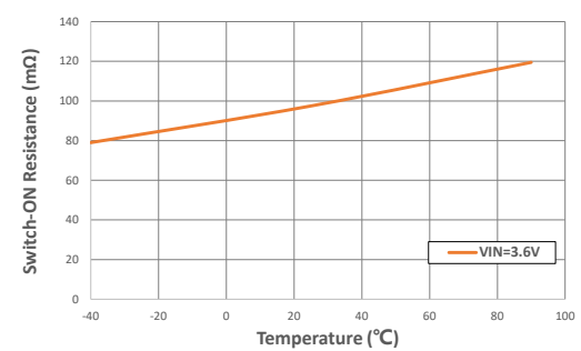
NMOS 导通电阻 vs. 温度
