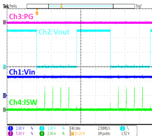
输出短路保护 / 恢复 ( V_{IN}=2.5V )
