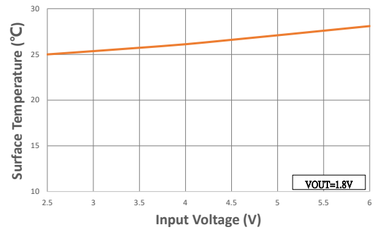
输出短路 表面温度 vs. 输入电压 (SOT23-5)
