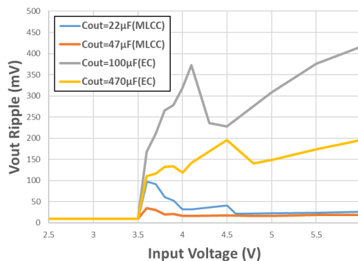
图 1. 输出纹波 VS. 输入电压
