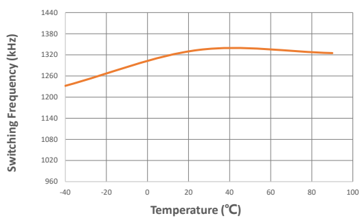
fsw vs. 温度
