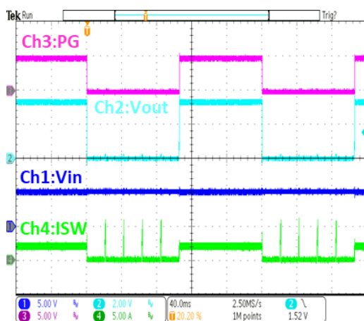
输出短路保护 / 恢复 ( V_{IN}=5V , I_{OUT}=2A )
