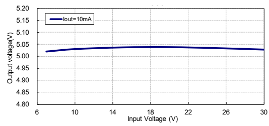
输出电压与输入电压：HT7550-1
