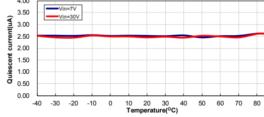
静态电流与温度：HT7550-1 ( I_{OUT} = 0mA )
