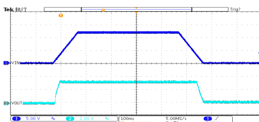
开关响应: HT7533-1 ( V_{IN}=12V , I_{OUT}=100mA , TRISE=TFALL=100ms )
