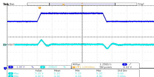
线性瞬态响应: HT7550-1 ( V_{IN}=6V\sim7V , I_{OUT}=10mA )
