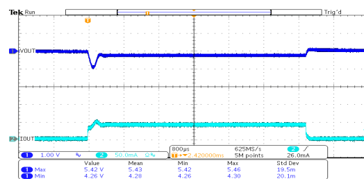
负载瞬态响应： HT7550-1 ( V_{IN} = 7V , I_{OUT} = 0mA \sim 40mA )
