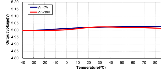
输出电压与温度：HT7550-1
