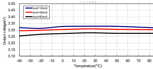
输出电压与温度：HT7533-1
