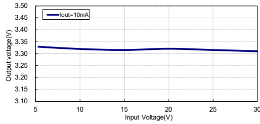
输出电压与输入电压：HT7533-1
