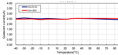
静态电流与温度：HT7533-1 ( I_{OUT} = 0mA )
