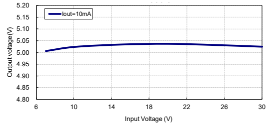
输出电压与输入电压：HT7550-3
