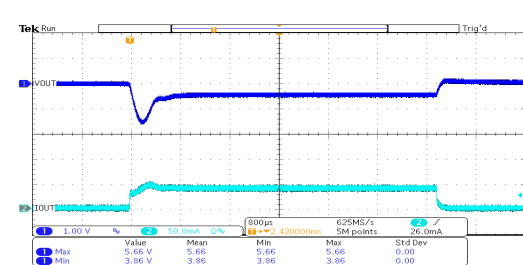
负载瞬态响应： HT7550-3 ( V_{IN} = 7V , I_{OUT} = 0mA \sim 40mA )
