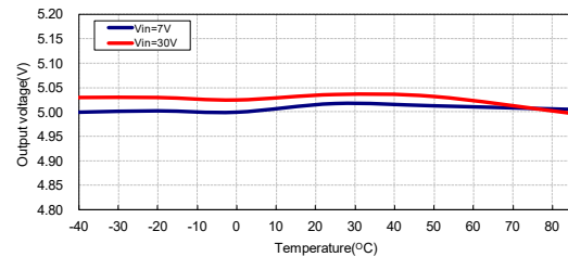
输出电压与温度：HT7550-3
