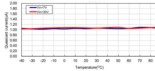
静态电流与温度：HT7550-3 ( I_{OUT} = 0mA )
