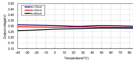
输出电压与温度：HT7533-3
