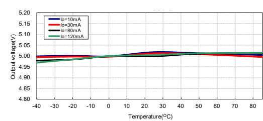
输出电压与温度：HT7550-3
