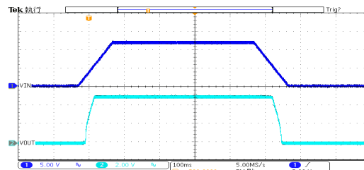
开关响应: HT7550-3 ( V_{IN}=12V , I_{OUT}=100mA , TRISE=TFALL=100ms )
