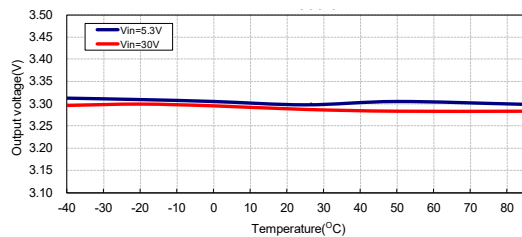
输出电压与温度：HT7533-3
