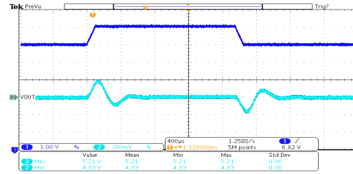
线性瞬态响应: HT7550-3 ( V_{IN}=6V\sim7V , I_{OUT}=10mA )
