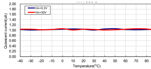
静态电流与温度：HT7533-3 ( I_{OUT} = 0mA )
