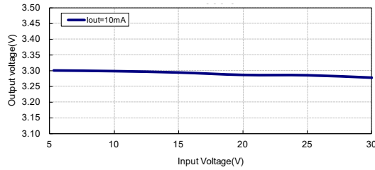
输出电压与输入电压：HT7533-3
